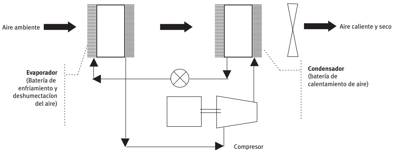
Fig. 61: Bomba de calor para el secado de aire en piscinas
