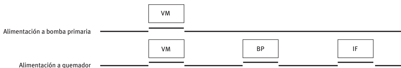
Fig. 35: Enclavamientos eléctricos
