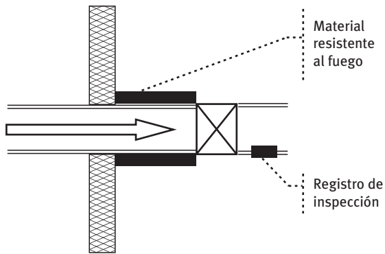
Fig. 82: Compuerta cortafuegos
